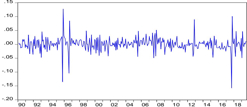
Gráfica 4.5 Primera diferencia del logaritmo de producción de gas natural 1990.1-2019.8
